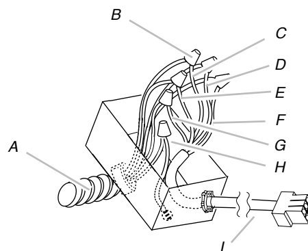
A. Conducto de cableado de 1/2" aprobado por UL o por CSA B. Conectores aprobados por UL C. Cables negros D. Cables blancos E. Cables rojos
