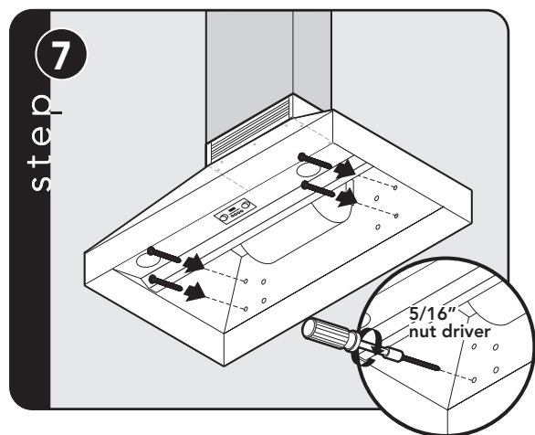
step 7 CAUTION: Secure vent hood. Make sure mounting screws are secured into framing. Use additional mounting screws and wall anchors, if necessary. ( MISE EN GARDE : Fixer solidement la hotte d'aération. S'assurer que les vis de fixation sont fixées solidement au cadrage. Utiliser des vis de fixation et chevilles murales additionnelles, si nécessaire.)
