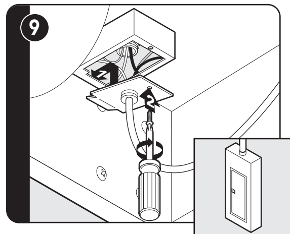
step 9 Replace electrical box cover. Make connection to breaker box. (Remplacer le couvercle du boîtier électrique. Faire les raccords à la boîte de disjoncteur.)
