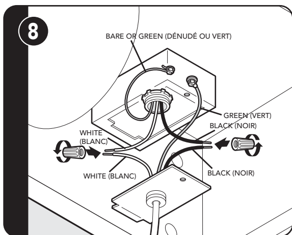
step 8 Connect black to black, white to white, and the green/bare wire under the green screw. NOTE: Housing wiring must be properly installed for wiring to be correct when wiring unit. (Raccorder le fil noir au noir, le blanc au blanc et le fil vert/dénudé sous la vis verte. NOTE : Le câblage du boîtier doit être correctement installé afin que le câblage soit adéquat lors du câblage de l'unité.)
