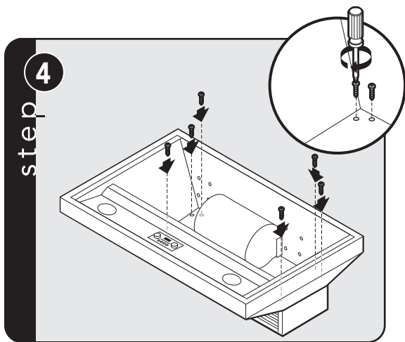
step 4 Attach with screws. (Fixer avec des vis.)
