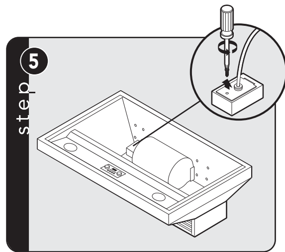
step 5 Remove electrical box cover. (Retirer le couvercle de boîtier électrique.)
