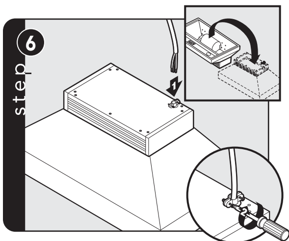
step 6 Flip hood over. Insert 6" of electrical wiring through the top of vent hood and secure. Refer to local codes. (Retourner la hotte. Insérer 6 po de câblage électrique par le haut de la hotte d'aération et fixer solidement. Reportez-vous aux codes locaux.)
