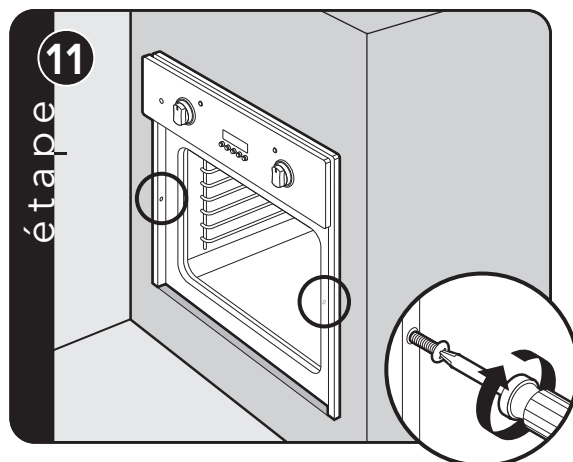
Posez des vis sur le côté du châssis. Remarque: 3 vis pour les fours simples, 4 pour les doubles (vis fournies)
