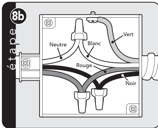
Option de câblage 2* (branchez le blanc sur le neutre d'arrivée, et le rouge sur le boîtier de raccordement relié à la terre)
